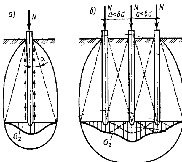
Рис. 6.18. Схемы передачи нагрузки на грунт основания:
