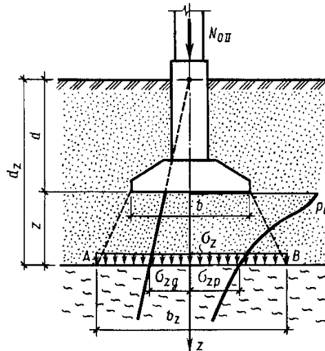
Рис. 2.19. Расчетная схема к проверке давления на подстилающий слой слабого грунта.
