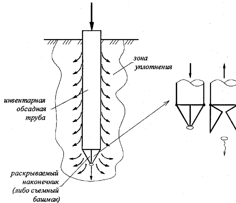
Рис. 6.16. Схема сваи Страуса
