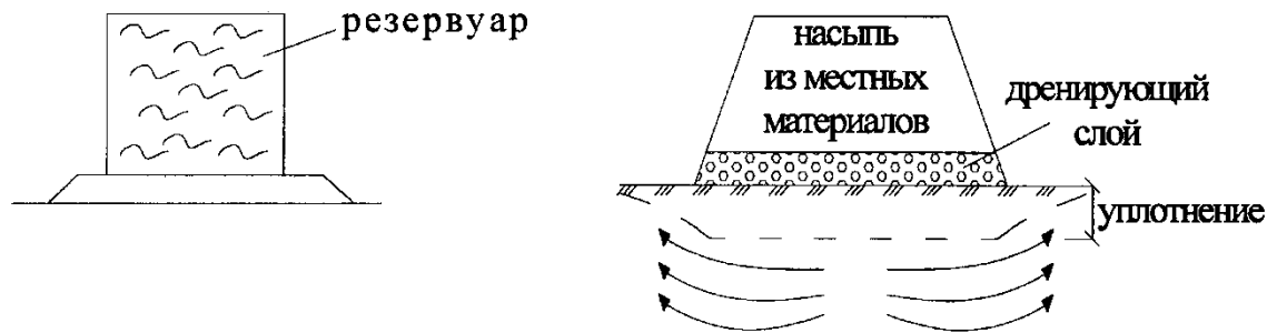
Рис. 4.17. Схема уплотнения статической нагрузкой
