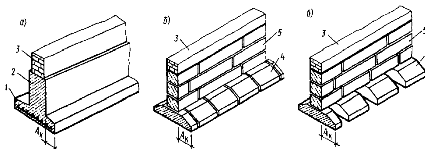
Рис. 2.6. Ленточные фундаменты:
