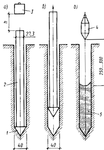
Рис.4.13. Схема устройства грунтовых свай способом сердечника:
