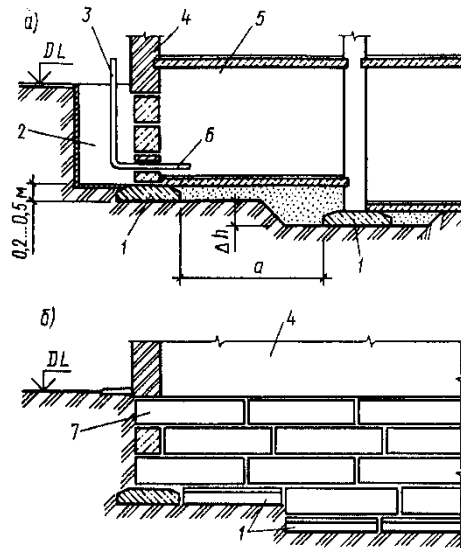
Рис. 2.12. Выбор глубины заложения фундамента в зависимости от конструктивных особенностей сооружения:
