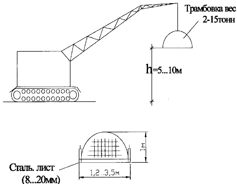
Рис. 4.7. Тяжелые трамбовки
