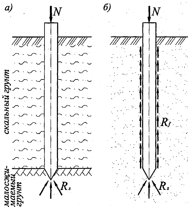
Рис.6.3. Схемы передачи нагрузки сваями на грунты основания: а – сваи-стойки ; б – висячие сваи
