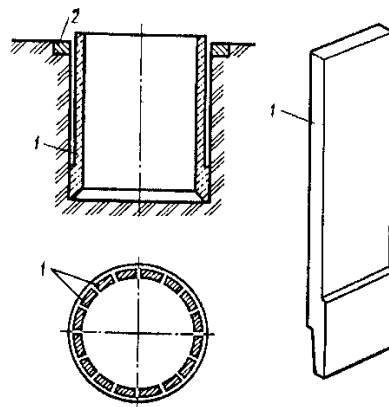
Рис. 5.5. Сборный опускающий колодец из вертикальных панелей:
