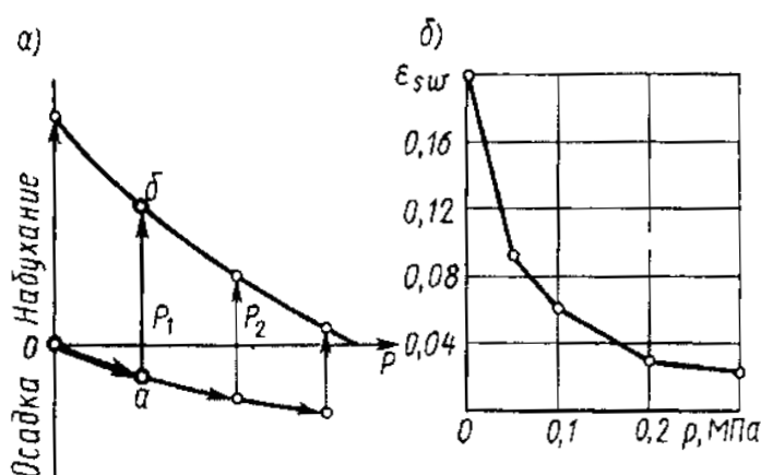
Рис. 7.3. Зависимости деформации набухающего грунта (а) и относительного набухания (б) от нормального давления
