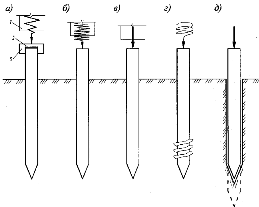
Рис. 6.12. Способы погружения свай:
