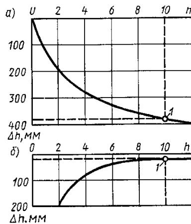
Рис. 4.5. Понижение уплотняемой поверхности в зависимости от числа ударов (проходов): а - от общего числа ударов; б - от каждых двух ударов; 1 - точка уплотнения до отказа
