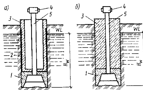
Рис.5.11. Схема устройства кессона:
