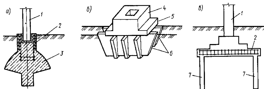
Рис. 2.5. Буробетонные (а), щелевые (б) и анкерные (в) фундаменты: 1 – колонна; 2 – арматурный каркас; 3 – фундамент; 4 – подколонник; 5 – плитная часть; 6 – бетонные пластины; 7 – анкеры (бурабивные сваи) d=15-20\text{см} , l=3-4\text{м} .
