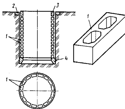
Рис. 5.4. Сборный опускной колодец из пустотелых прямоугольных блоков:
