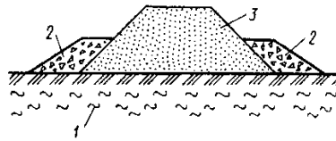
Рис. 4.3. Увеличение устойчивости насыпи на слабых грунтах методом боковой пригрузки:
