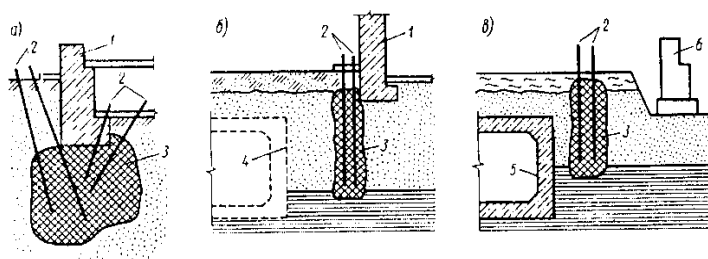
Рис. 4.21. Схема закрепления методом силикатизации оснований фундаментов (а), защиты фундаментов зданий при строительстве подземных сооружений (б), при возведении зданий (в):
