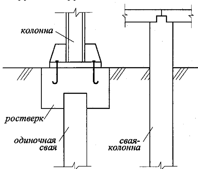
Рис. 6.4. Схемы одиночной сваи и сваи-колонны
