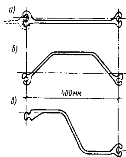
Рис. 3.3. Профили прокатного стального шпунта:
