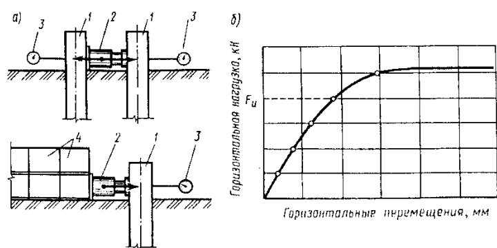
Рис. 6.22. Испытания свай горизонтальной нагрузкой:
