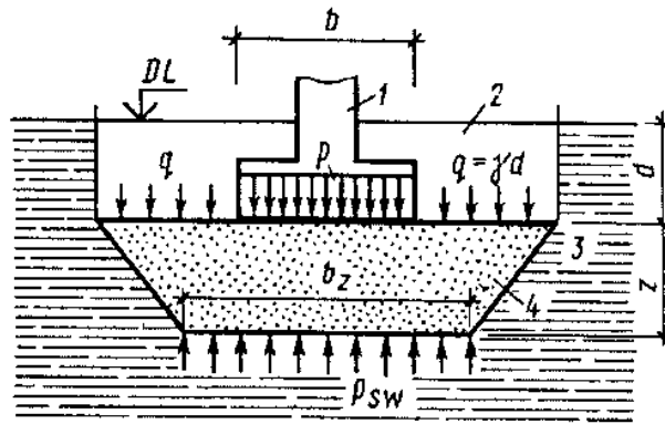
Рис. 7.4. Схема сил, действующих на компенсирующую подушку: 1 – фундамент; 2 – обратная засыпка; 3 – набухающий грунт; 4 – песчаная компенсирующая подушка.
