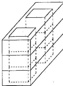
Рис. 5.6. Схема расположения пустот в блоках опускающего колодца
