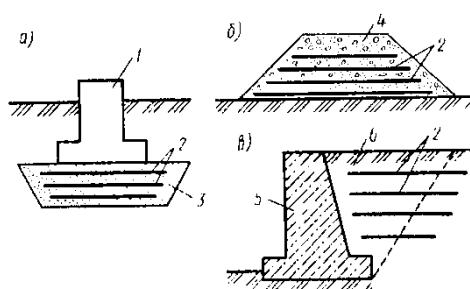
Рис. 4.2. Армировании грунта в искусственном основании фундамента (а), при устройстве насыпи (б), при воздействии засыпок (в):
