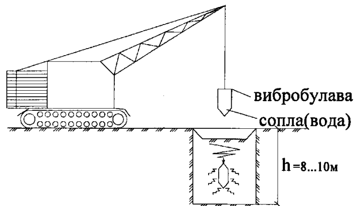
Рис. 4.16. Схема уплотнения вибробулавой
