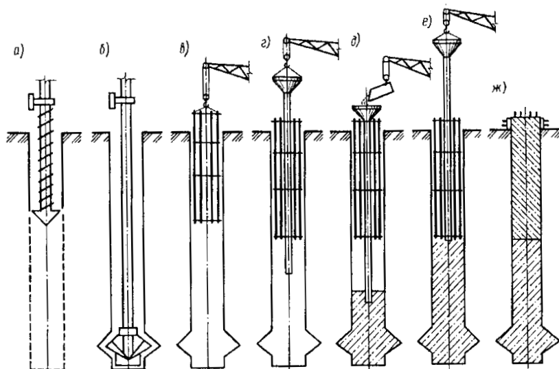
Рис.6.14. Последовательность изготовления буронабивных свай без оболочек:
