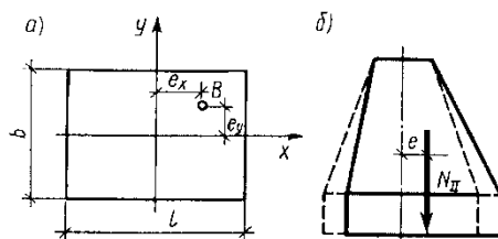
Рис. 2.17. внецентренное нагружение фундамента относительно двух главных осей инерции:
