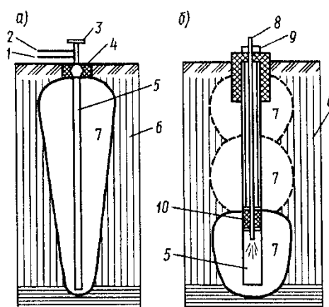
Рис. 4.22. Схемы термического закрепления грунтов при сжигании топлива в устье скважины (а) и при передвижении камеры сгорания вдоль скважины (б):
