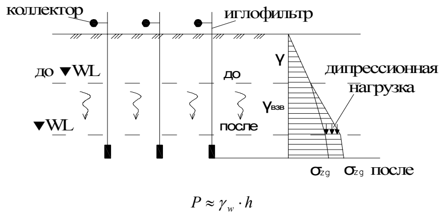
Рис. 4.19. Схема уплотнения грунтов с помощью водопонижения иглофильтрами
