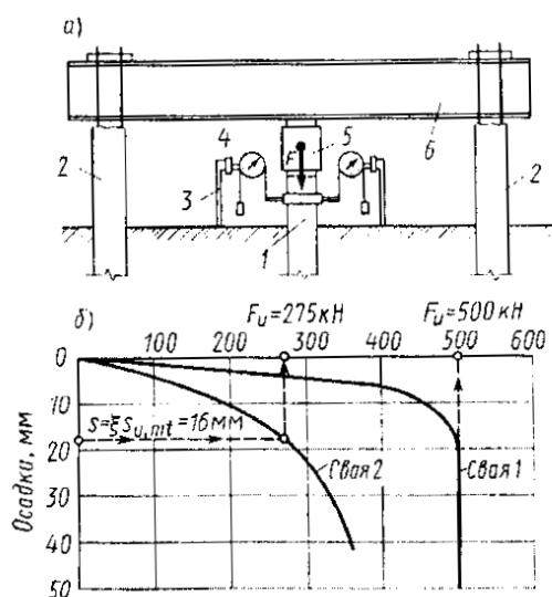
Рис. 6.19. Испытание свай вертикальной статической нагрузкой:
