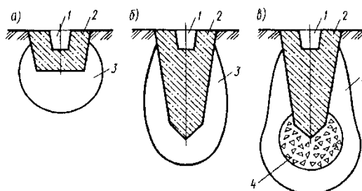
Рис. 4.10. Схемы устройства методом вытрамбовывания котлованов фундаментов с плоской подошвой (а), с заостренной подошвой обычного типа (б) и с уширенным основанием (в):
