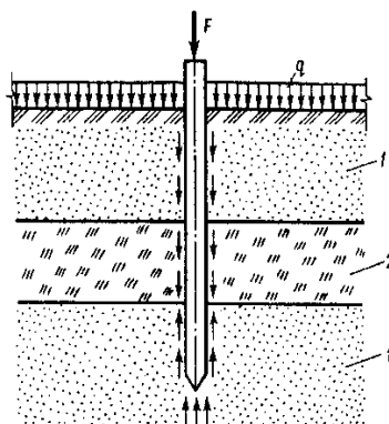
Рис. 6.21. Развитие отрицательных сил трения на боковой поверхности сваи:
