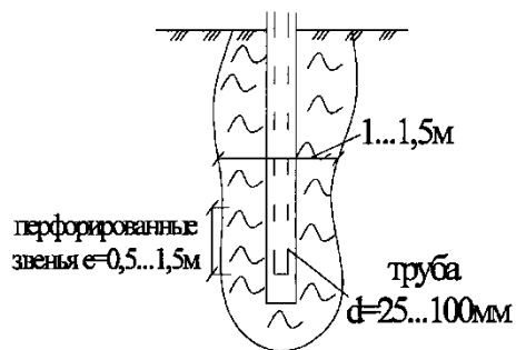
Рис. 4.20. Схема цементации
