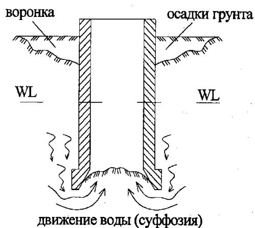
Рис. 5.7. Схема движения воды
