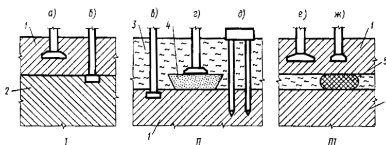
Рис. 2.10. Схемы напластований грунтов с вариантами устройства фундаментов:
