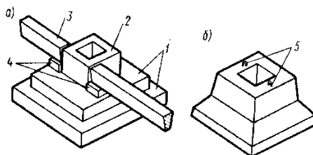
Рис. 2.4. Сборный фундамент под колонну:
