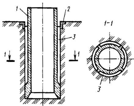
Рис.5.9. Схема погружения опускного колодца в тиксотропной рубашке:
