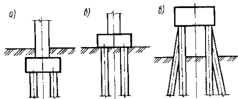
Рис.6.1. Типы свайных ростверков: а, б – низкий; в – высокий
