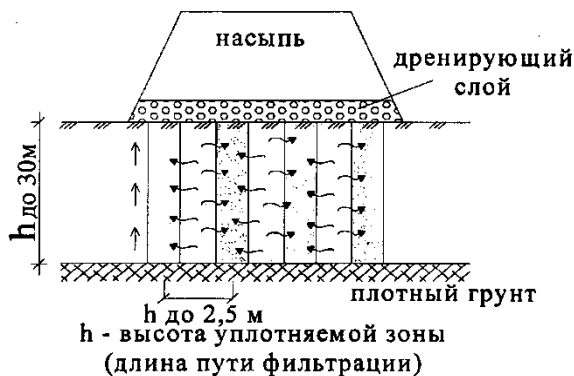
Рис. 4.18. Схема уплотнения грунтов с помощью вертикальных дрен
