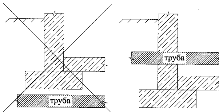
Рис. 2.13. Схема неправильного и правильного ввода коммуникаций
