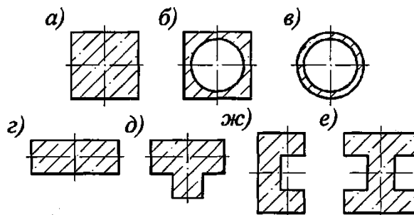
Рис. 6.9. Сечения железобетонных свай:
