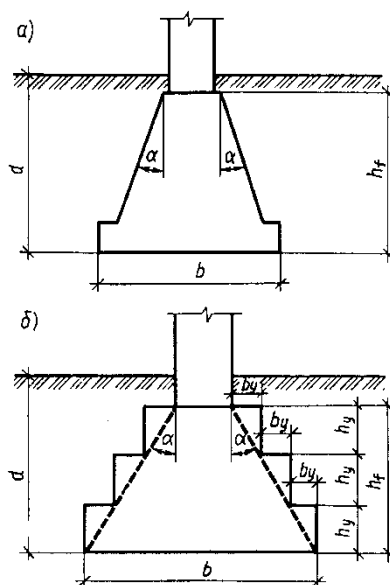
Рис. 2.3. Конструкция жесткого фундамента:
