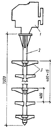
Рис. 4.15. Схема виброустановки ВУУП – 6:
