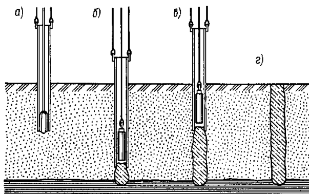
Рис. 6.17. Последовательность изготовления свай Страуса:
