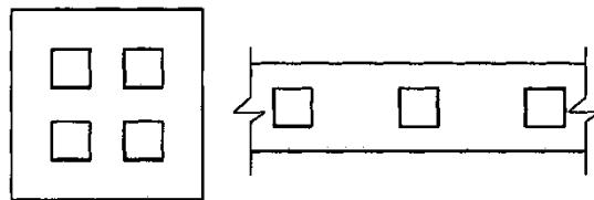
Рис. 6.2. План ростверка
