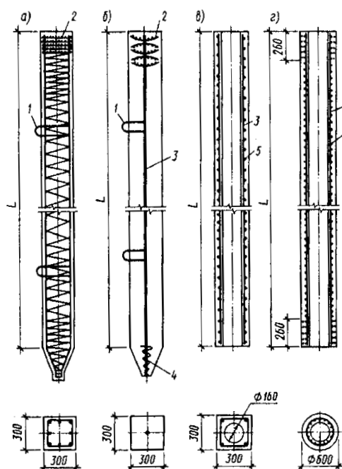
Рис. 6.11. Конструкция железобетонных свай:
