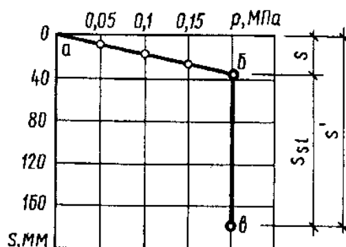
Рис. 7.1. Осадка фундамента на лессовом грунте
