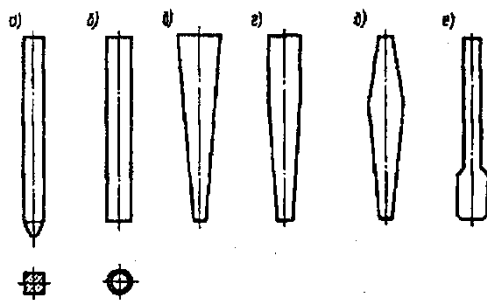
Рис. 6.10. Железобетонные сваи различного профиля:
