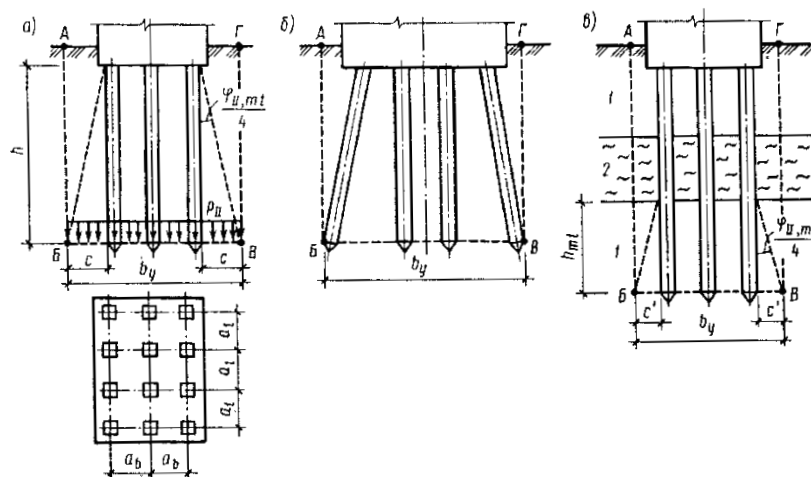
Рис. 6.25. Схемы условных фундаментов для расчета по второй группе предельных состояний
