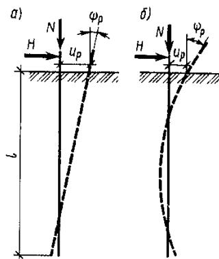
Рис. 6.23. Схемы работы горизонтально нагруженных свай
