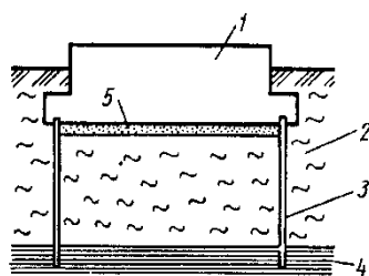
Рис. 4.1. Усиление основания с помощью шпунтового ограждения:
