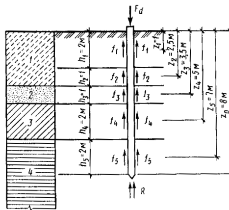
Рис. 6.20. Расчетная схема к определению несущей способности сваи практическим методом
