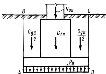
Рис. 2.14. Расчетная схема центрально нагруженного фундамента.
