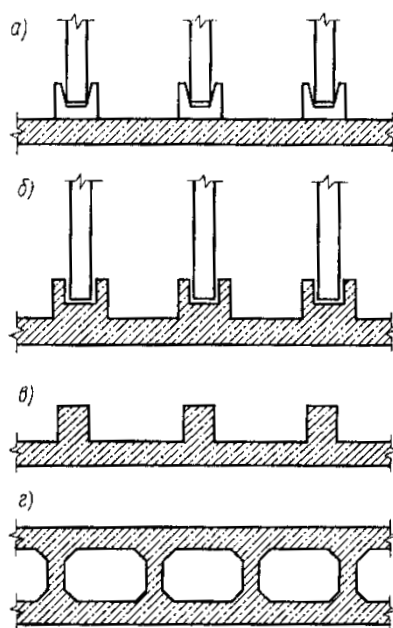
Рис. 2.8. Сплошные фундаменты:
