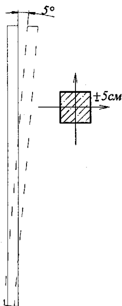
Рис. 6.5. Схема максимальных допустимых горизонтальных и вертикальных отклонений при погружении одиночной сваи
