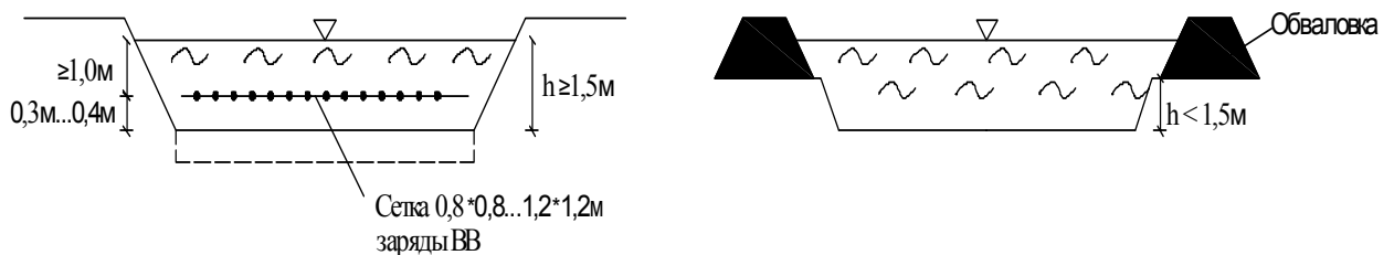
Рис. 4.9. Схема уплотнения рыхлых песчаных грунтов подводными взрывами
