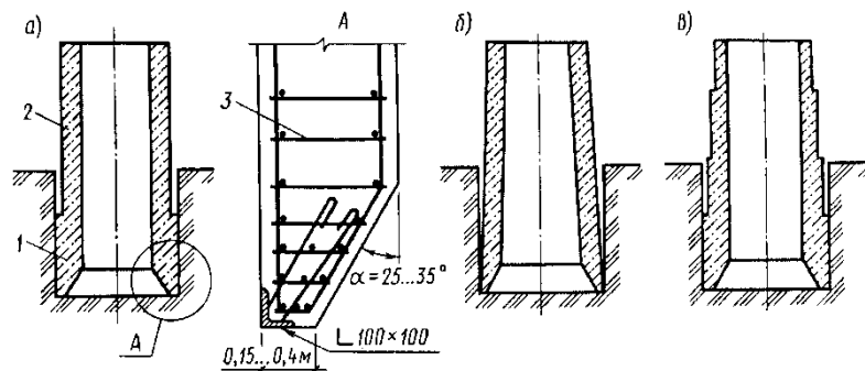
Рис. 5.3. Форма вертикальных сечений монолитных опускных колодцев:
