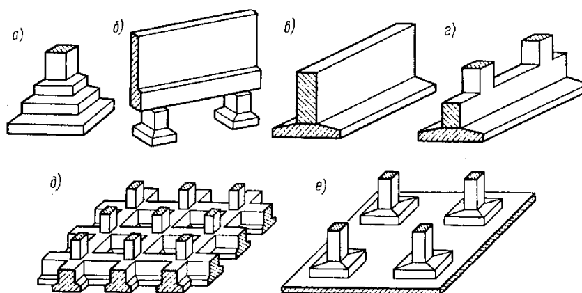
Рис. 2.2. Основные типы фундаментов мелкозаложеная:
