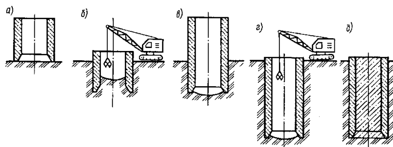
Рис. 5.1. Последовательность устройства опускного колодца:
