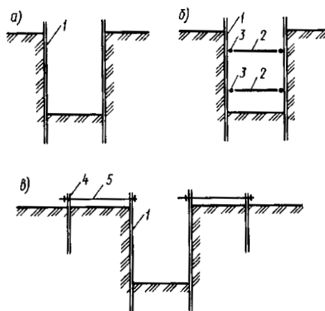
Рис. 3.4. Схемы шпунтовых ограждений:
