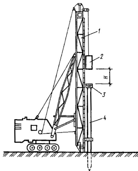
Рис. 6.13. Забивка свай механическим молотом:
