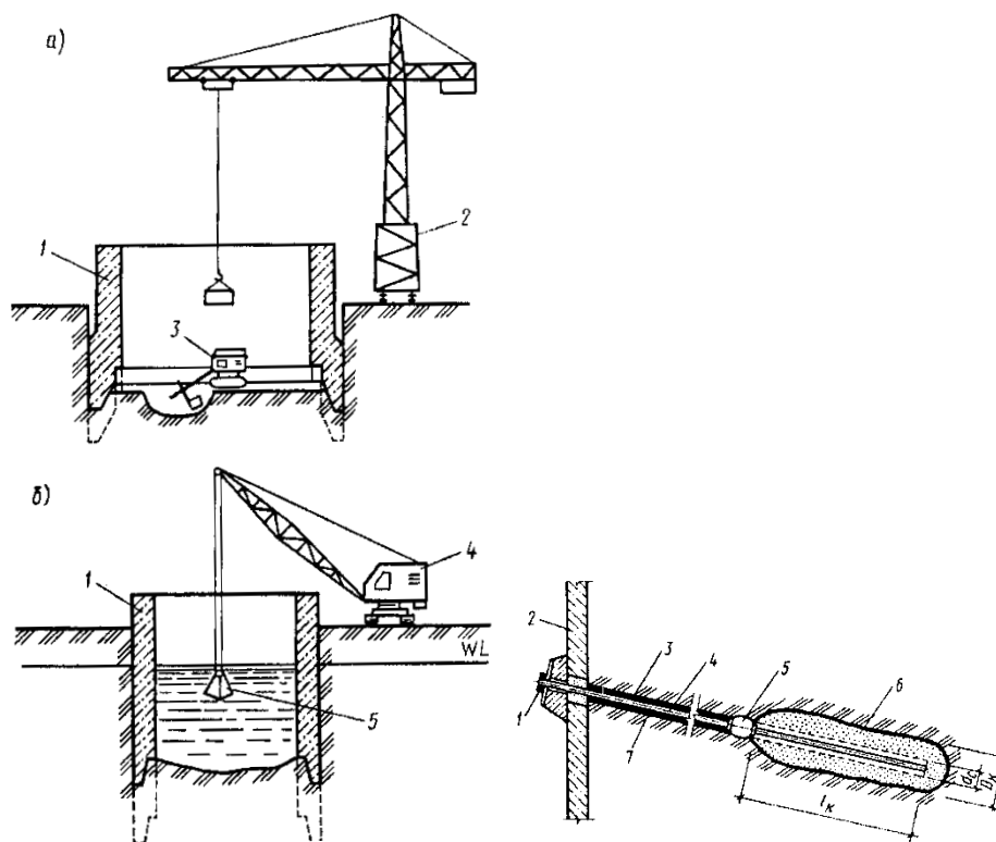
Рис.5.8. Разработка грунта в опускном колодце:
