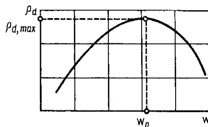
Рис. 4.4. Зависимость плотности скелета уплотняемого грунта от влажности при стандартном уплотнении
