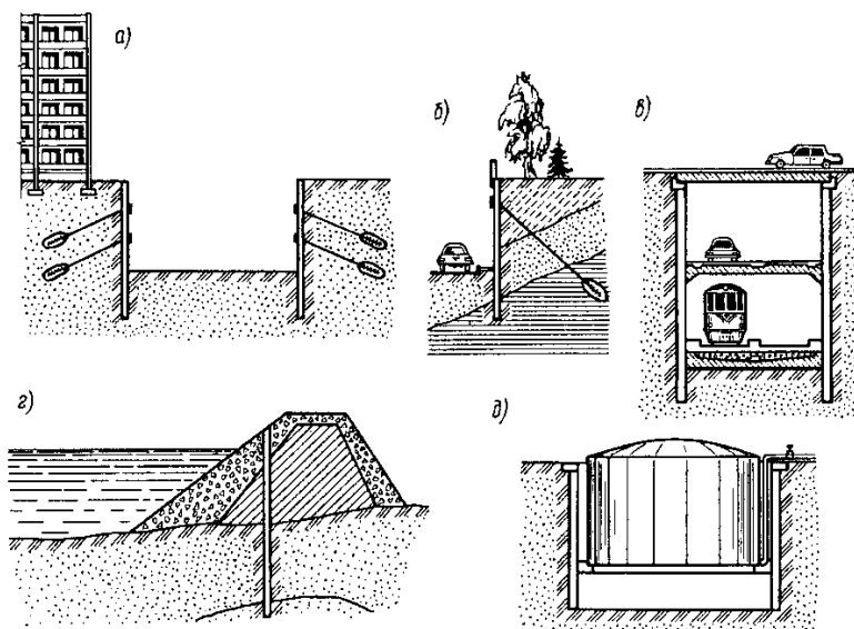
Рис. 5.12. Конструкции, сооружаемые способом «стена в грунте»: а – котлованы в городских условиях; б – подпорные стенки; в – тоннели; г – противодиффузионные диафрагмы; д – подземные резервуары
