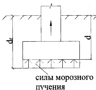
Рис. 2.11. Схема морозного пучения основания
