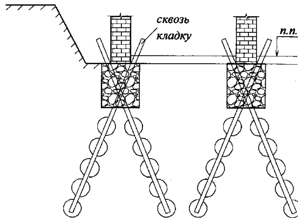
Рис. 6.15. Схема буринъекционных свай
