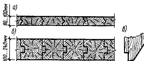
Рис. 3.2. Деревянное шпунтовое ограждение:
