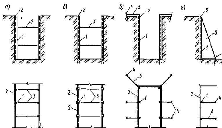
Рис. 3.1. Крепление вертикальных стенок выемок:
