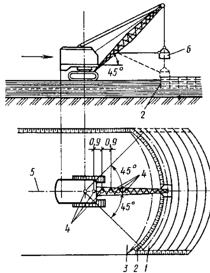
Рис. 4.8. Схема поверхностного уплотнения грунта тяжелой трамбовкой.
